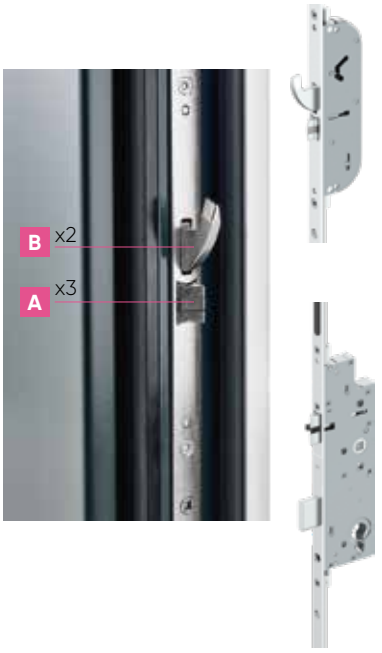
A 3 PÊNES 1/2 TOUR à archet facilitant l'entrée et la prise dans la gâche centrale.
