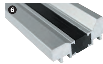
Seuil en aluminium à rupture de pont thermique (hauteur : 20 mm)
