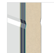
Remplissage panneaux acier et mousse isolante 40 mm
