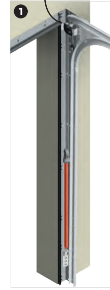
2 double-ressorts de traction intégrés dans les rails verticaux
