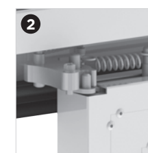
Train de double-roulettes et rail de guidage intégré au cadre en aluminium
